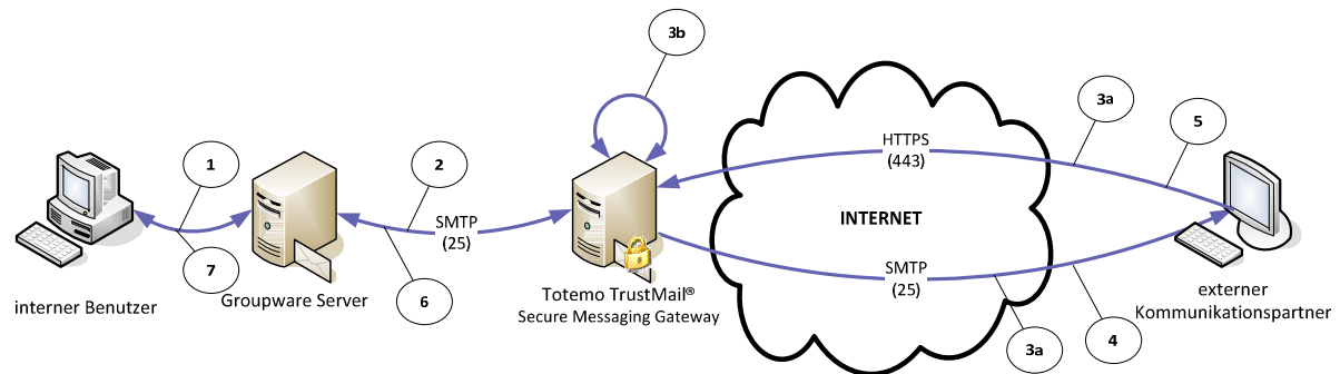
Abbildung 1 – Funktionsweise Totemo TrustMail® PushedPDF
